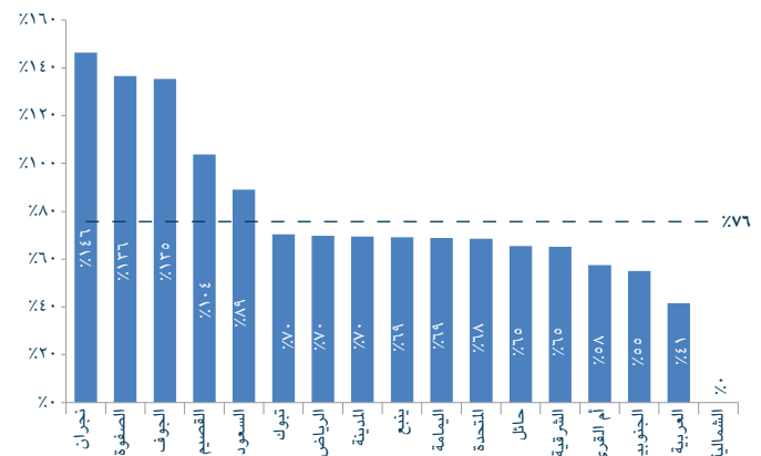
متوسط المبيعات/ إنتاج الكلنكر | الشركات
