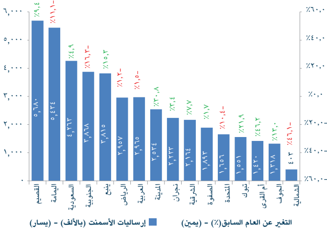
الشكل ٦: إرساليات الأسمت والكلنكر في أول ١١ شهر من ٢٠٢٤ (المبيعات المحلية بالآلاف طن)
