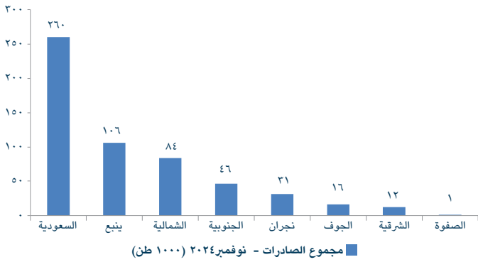
الشكل ٢: صادرات الأسمنت والكلنكر لشهر نوفمبر ٢٠٢٤ (ألف طن)
