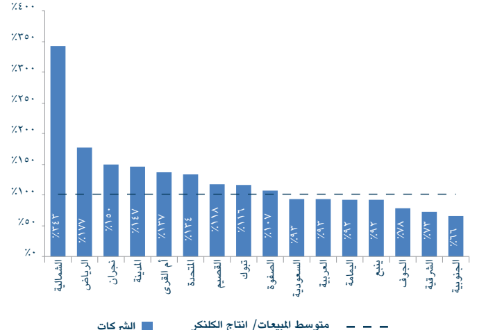
الشكل ٧: المبيعات إلى إنتاج الكلنكر لشهر نوفمبر ٢٠٢٤
