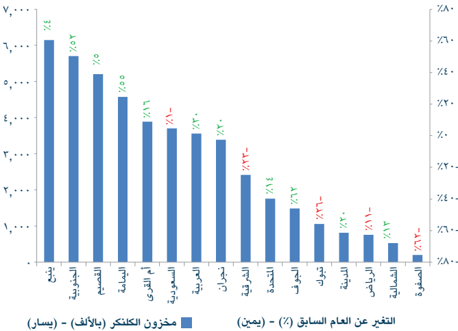
الشكل ٨: مخزونات الكلنكر - سبتمبر ٢٠٢٤ (بالآلاف)
