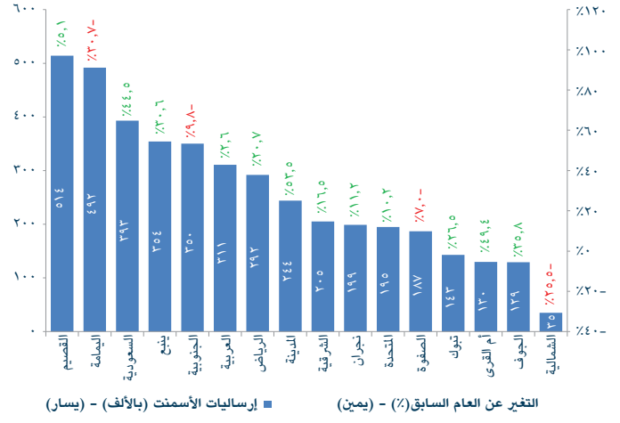
الشكل ٥: إرساليات الأسمنت والكلنكر خلال سبتمبر ٢٠٢٤ (المبيعات المحلية)
